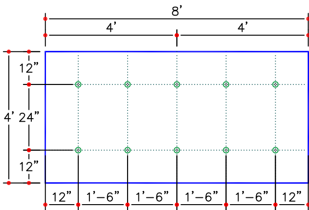
10 FASTENERS PER 4'X8' BOARD
