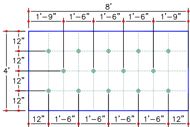
14 FASTENERS PER 4'X8' BOARD
