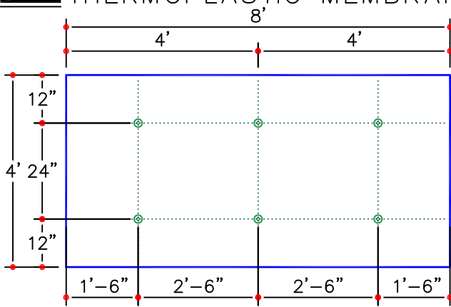
6 FASTENERS PER 4'X8' BOARD
