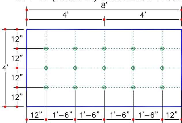
15 FASTENERS PER 4'X8' BOARD
