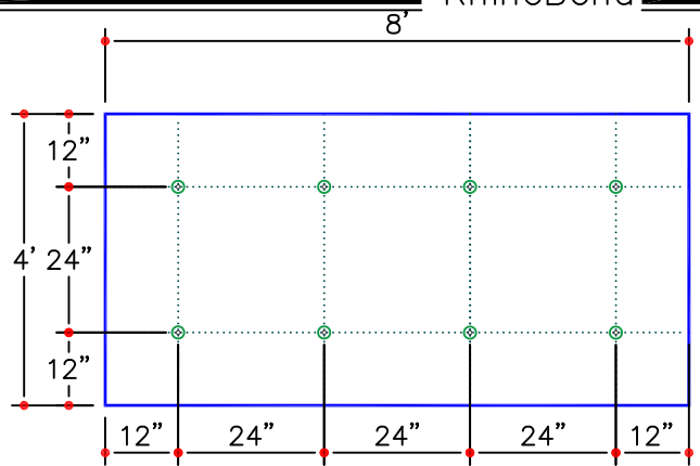
8 FASTENERS PER 4'X8' BOARD
