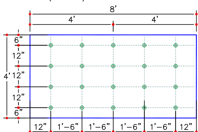
20 FASTENERS PER 4'X8' BOARD
